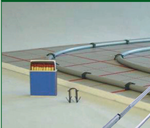
Sponkovací systém
