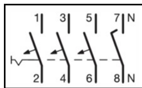
400 V napájanie
