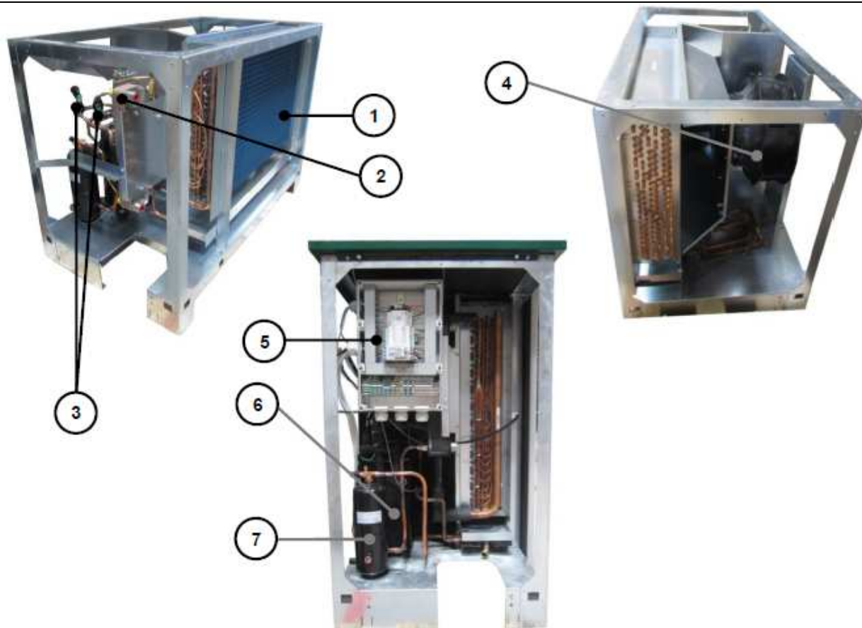
Obr.2.2: Pohľad na zariadenie bez opláštenia
