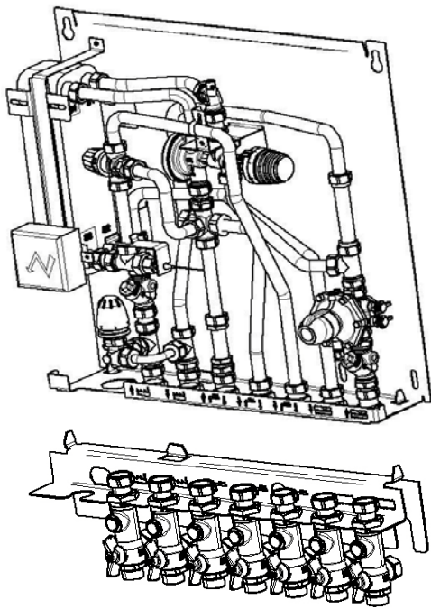
Výmenníková stanica – vyhotovenie na omietku
