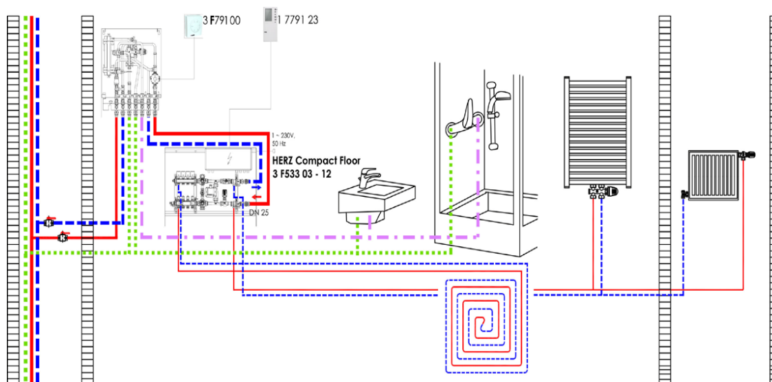
Vyhotovenie 3 F533 xx s 3-mi až 12-timi vykurovacími okruhmi pre podlahové vykurovanie a s dvoma okruhmi pre vykurovacie telesá paralelne napojené.
