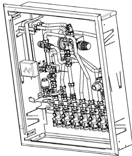
Výmenníková stanica – vyhotovenie pod omietku
