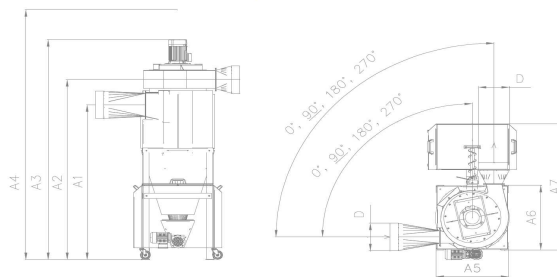
BM300-500
