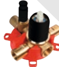
UH00368B Podomietkové teleso pre 2 odberné miesta
